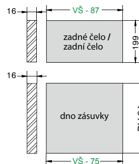
Rozměry zadního čela a dna zásuvky [mm] / Rozměry zadního čela a dna zásuvky [mm]
