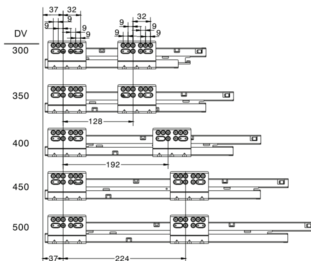
Rozměry zadního čela a dna zásuvky [mm] / Rozměry zadního čela a dna zásuvky [mm]
