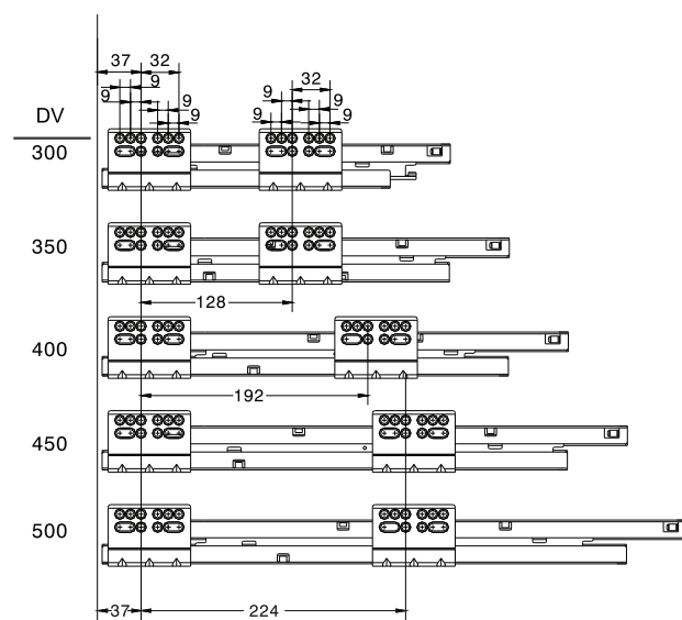
Montážny náčrt - vnútorná zásuvka s 1-relingom [mm] / Montážní náčrt - vnitřní zásuvka s 1-relingem [mm]
