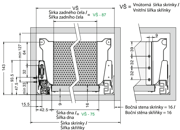
Rozměry zadného čela a dna zásuvky [mm] / Rozměry zadního čela a dna zásuvky [mm]
