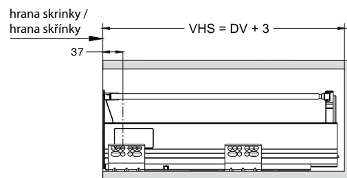
Montážny náčrt - vnútorná zásuvka s 1-relingom [mm] / Montážní náčrt - vnitřní zásuvka s 1-relingem [mm]
