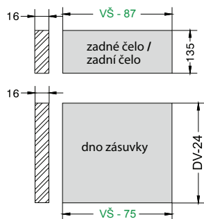
Rozměry zadného čela a dna zásuvky [mm] / Rozměry zadního čela a dna zásuvky [mm]
