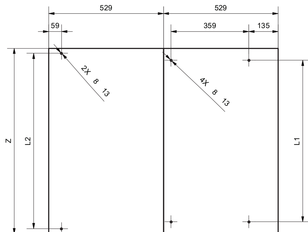
Pohľad zdola
