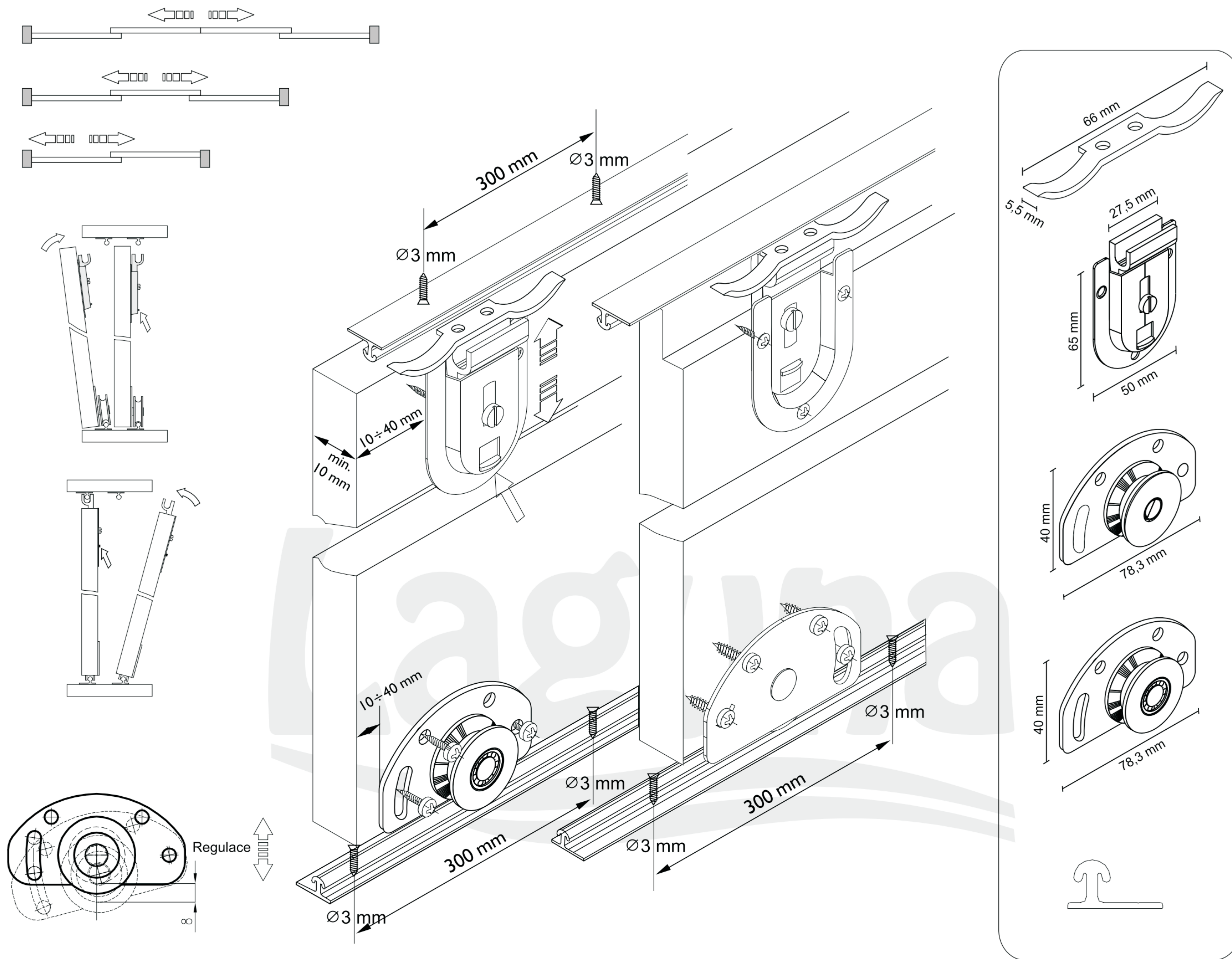
montáž kování uvnitř křídla
